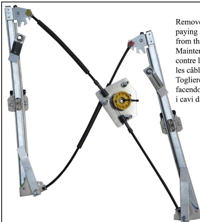
A POWER WINDOW LEFT ALZACRISTALLI ELETTRICO SX
