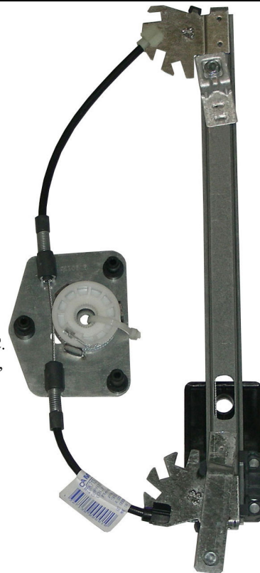
POWER WINDOW LEFT ALZACRISTALLI ELETTRICO SX
